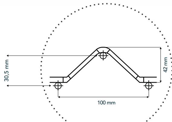
PLI DE LA GRILLE
