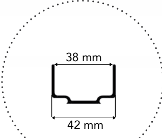
GUIDE PLAQUE (en option)
