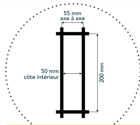
FIL HORIZONTAL ET VERTICAL 5 mm d'épaisseur
