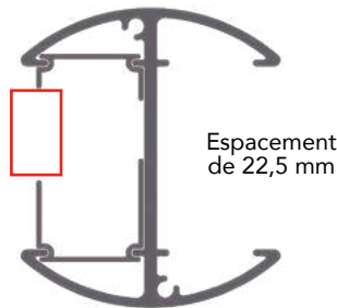
Exemple de combinaison N°9
