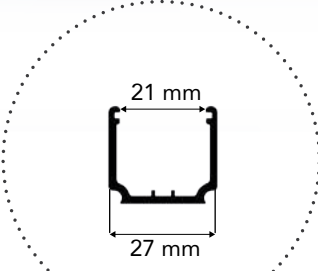
PROFIL UNIQUE (pour angle, finition et parcose en option)
