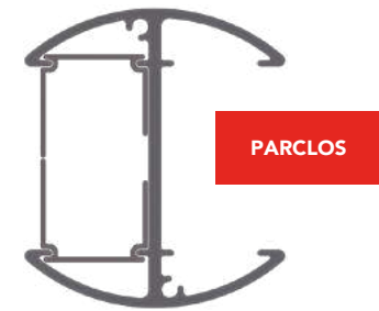
Exemple de combinaison N°15
