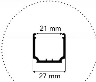
PROFIL UNIQUE (pour angle, finition et pardose en option)
